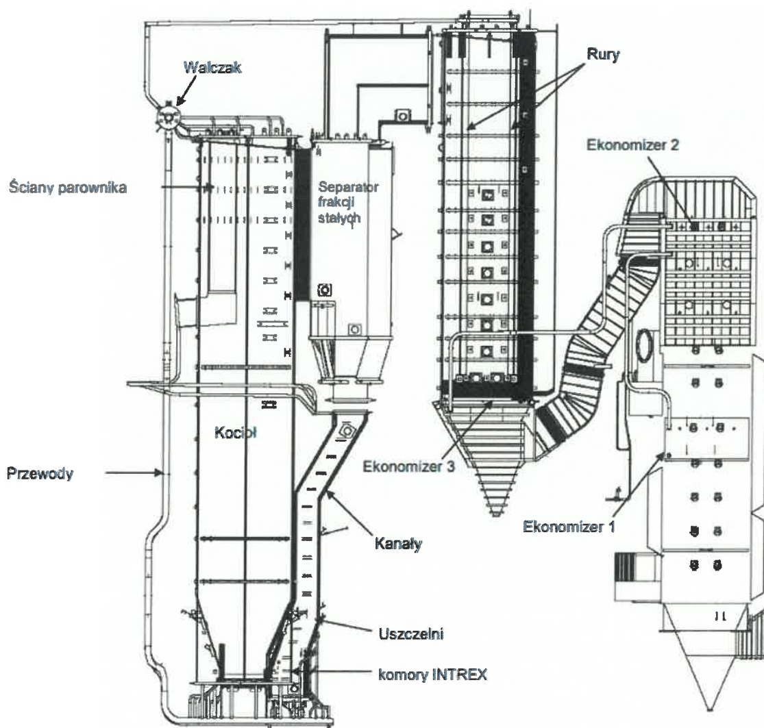
Rysunek 1. Kocioł, ekonomizer i parownik - Polaniec
