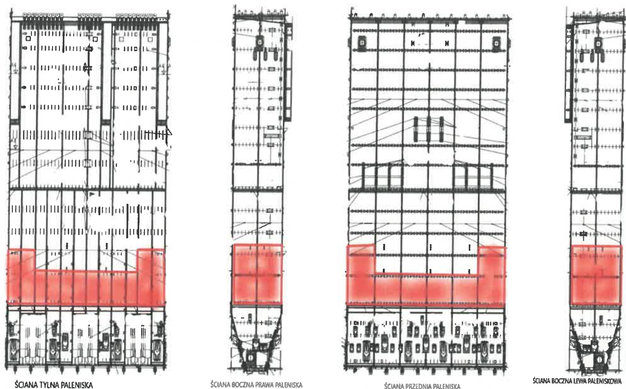
Rys. 2 Zakres powierzchni zabezpieczonych powłokami ochronnymi.
