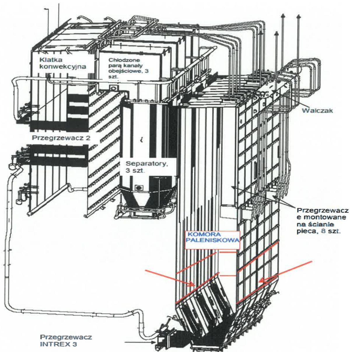
Rysunek 1. System kotła i przegrzewacza - Polaniec
